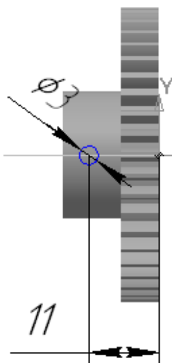
Рис. 24. Моделювання отвору під установчий гвинт
