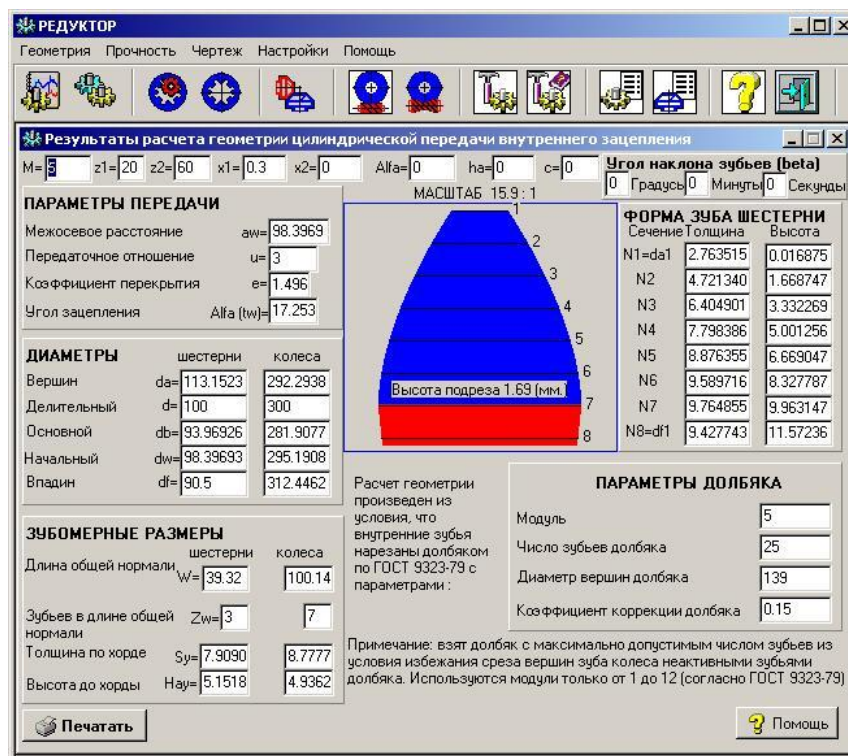
Рис. 2.18. Розрахунково-графічна робота «Розрахунок редуктора» з дисципліни «Робочі машини» виконується в програмі «Редуктор»
