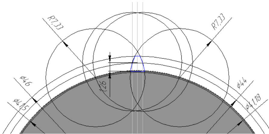
Рис. 12. Створення ліній побудови стилем ліній «Допоміжна»
